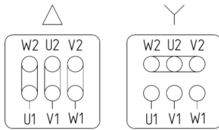
Рис. 15 Схема клеммных соединений
