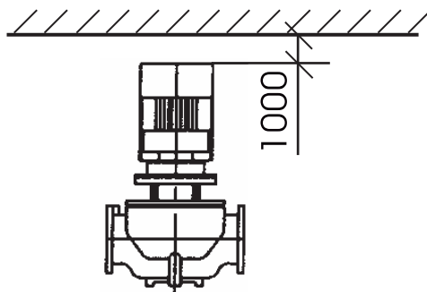
Рис 9 Электродвигатель \leq 4 кВт
