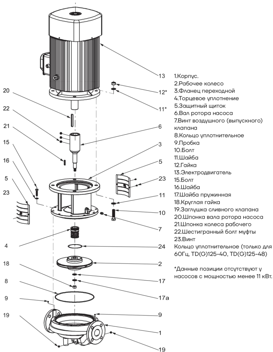
Рис. 18-А TD32-TD150
