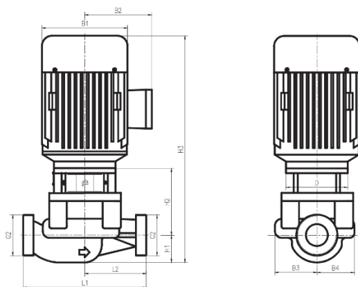
Рис. 20а. Габаритно-присоединительные размеры модели TD32-6(I)/2
